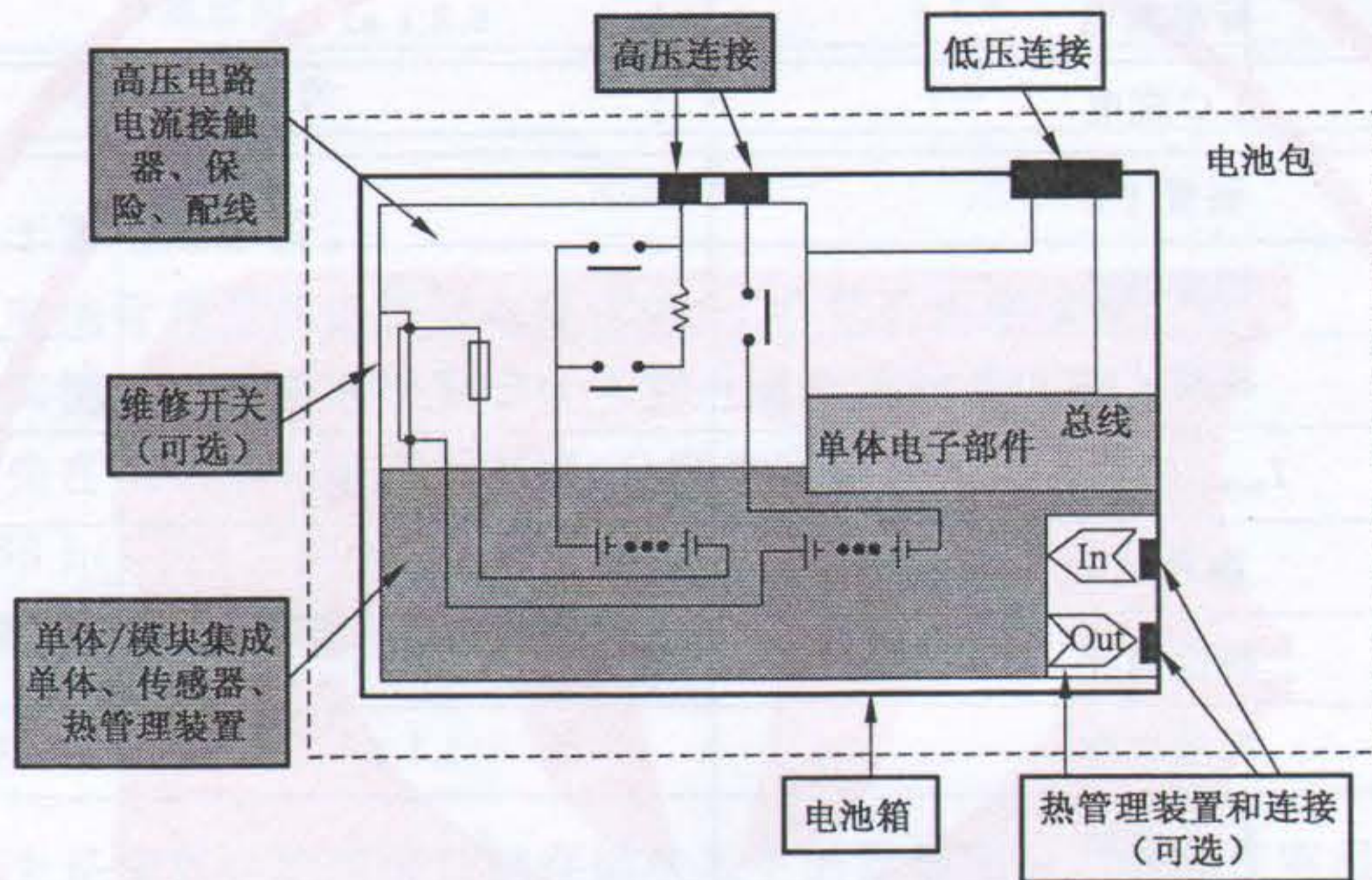
图 A.1 蓄电池包典型结构
