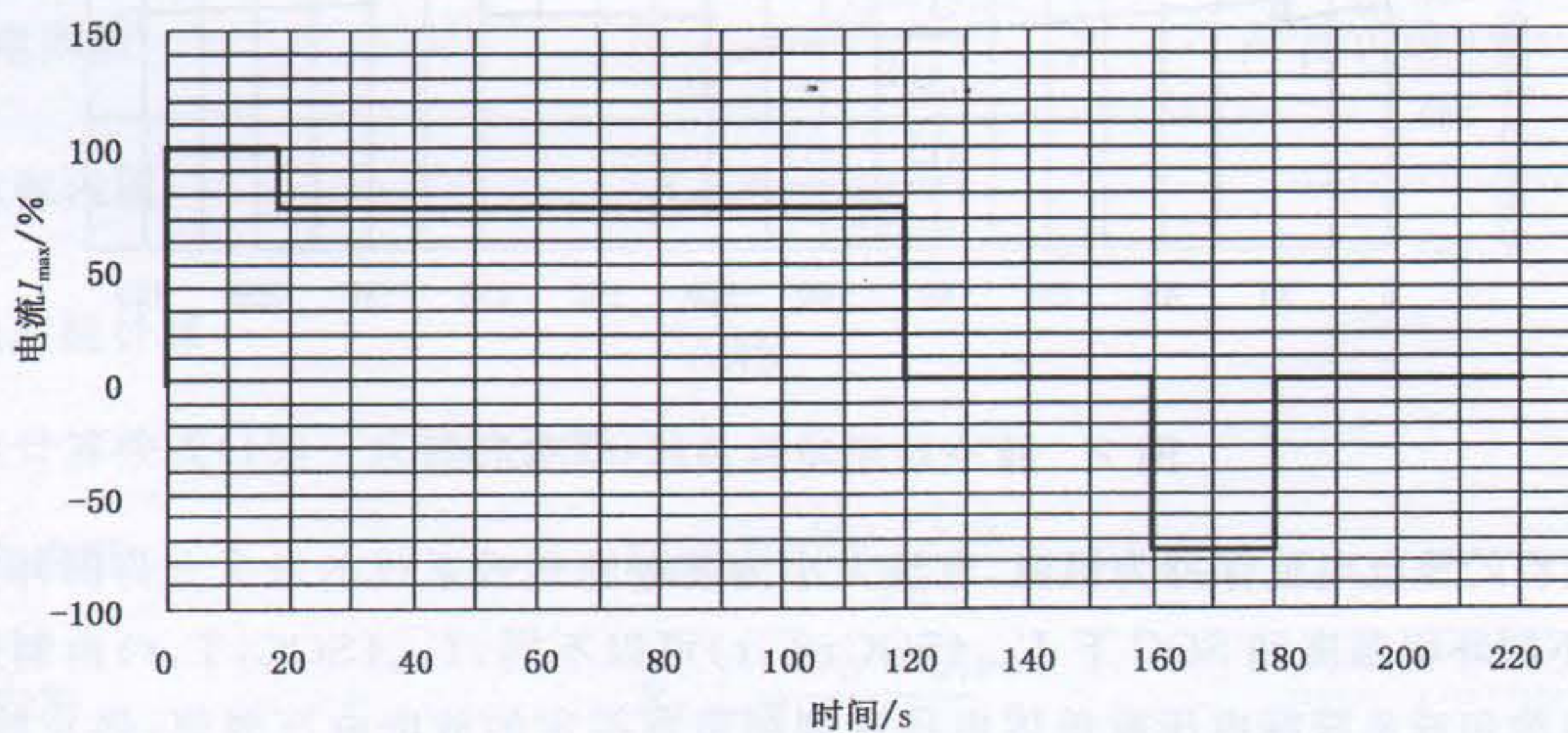
图 1 脉冲功率特性曲线-电流示例
