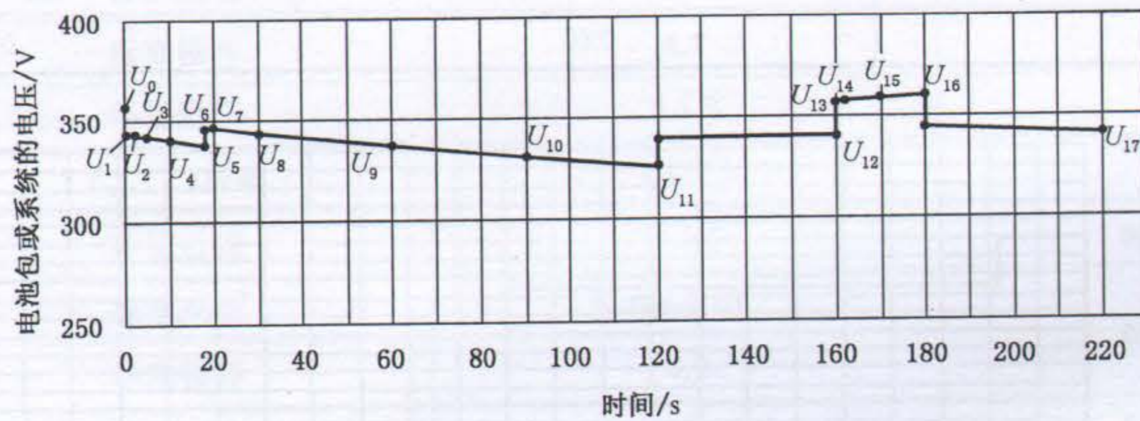
图 2 脉冲功率特性曲线-电压示例
